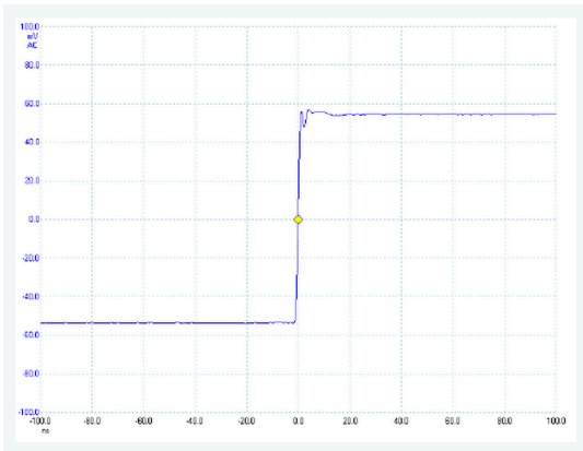
Abbildung 4: Gute Kompensation
