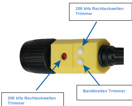
Abbildung 2: Frequenz Kompensation Trimmer
