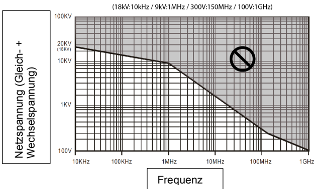
Abbildung 5: Derating Spannungskurve
