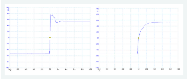
Abbildung 3: Über/Unter-Kompensation
