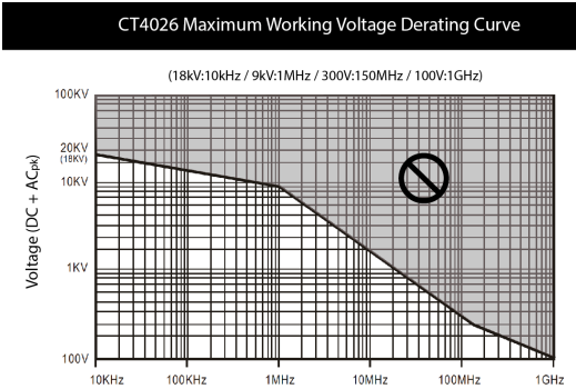
Figure 5: Courbe de limitation de la tension en fonction de la fréquence
